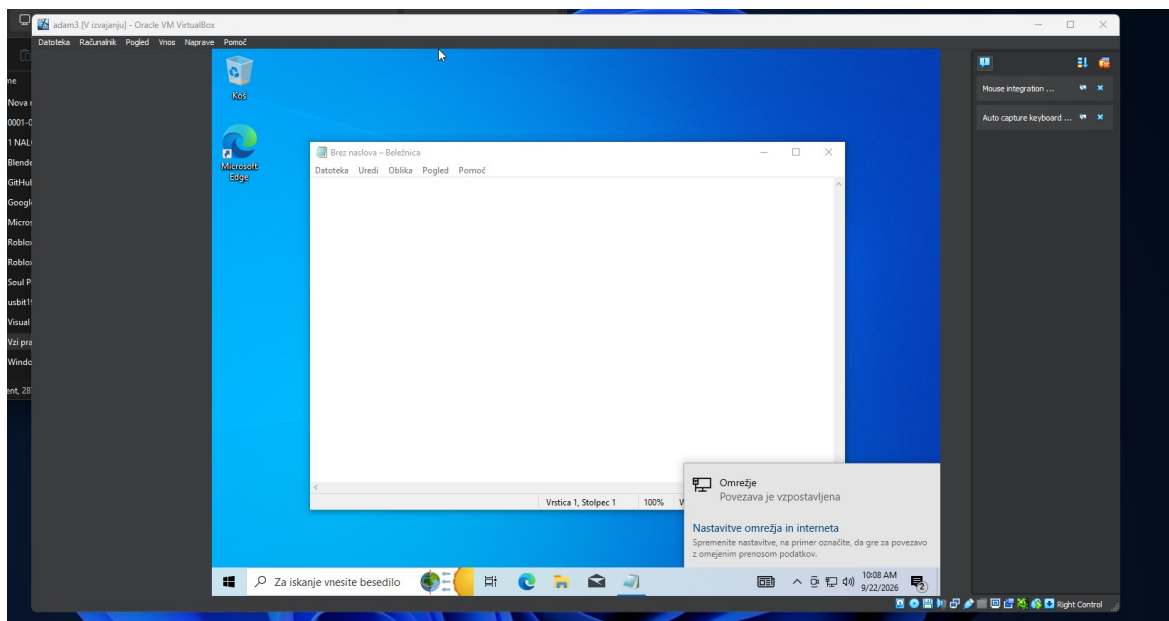
Slika 2: Preverjanje povezave
